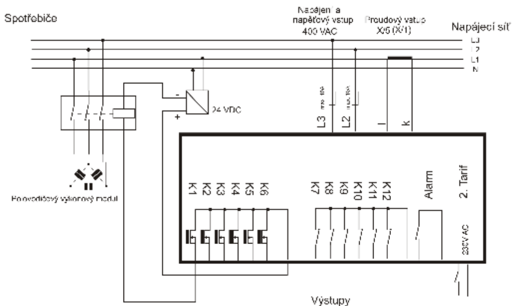
Obrázek 5. Schéma připojení regulátoru , kde v šestici jsou jen polovodičové stupně
