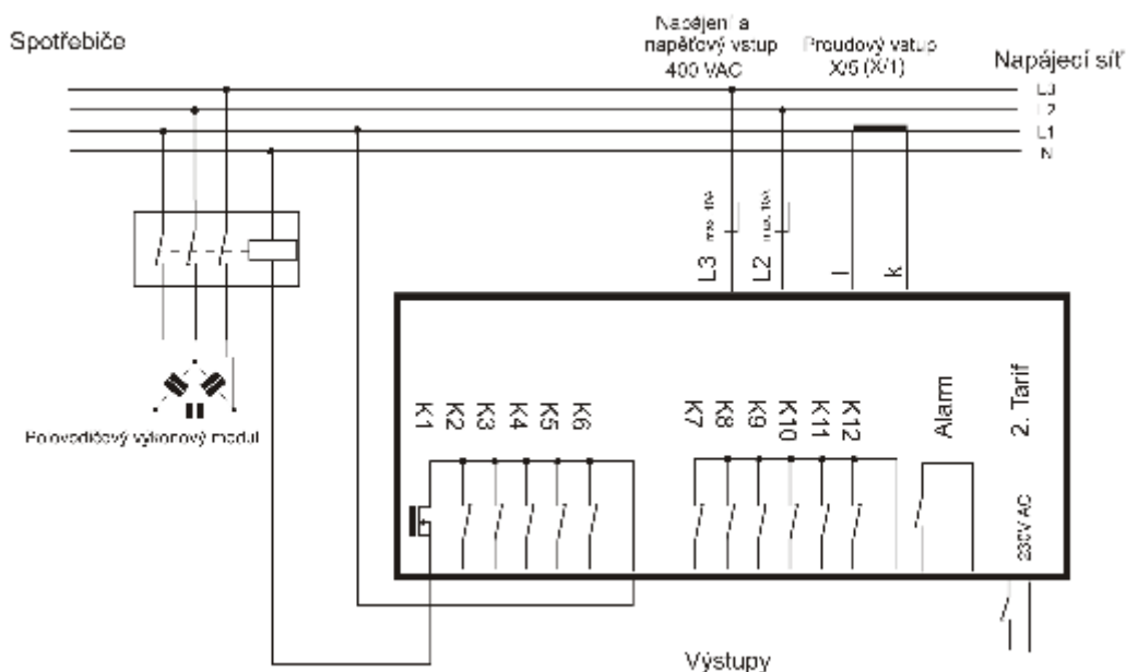
Obrázek 4. Schéma přípojení regulátoru s kombinací polovodičových a stykačových stupňů
