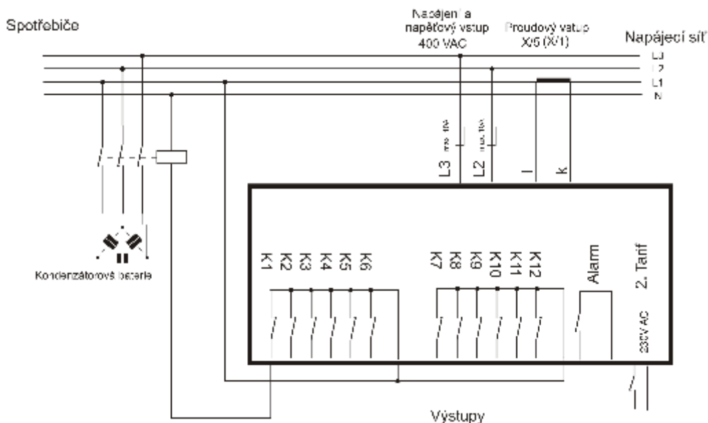
Obrázek 3. Schéma přípojení regulátoru pro stykačové stupně
